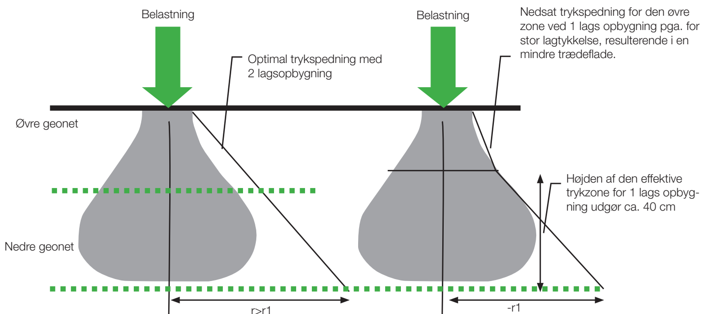
Figur 9 Belastningen fra enkeltkraften får ved store bærelagstykkelser mindre indvirkning på det nederste lag geonet - der kan opnås en yderligere trykspredningseffekt ved indbygning af flere lag geonet
