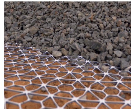
Tensar InterAx hexagonale geonet
