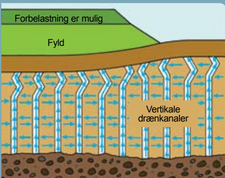
Med vertikaldræn
