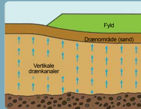
Uden vertikaldræn
